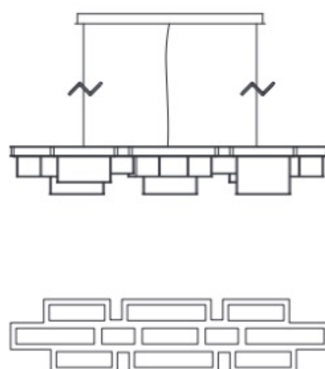
Item G01 L.135 x D.30 cm H.45 cm min - 138 cm max
