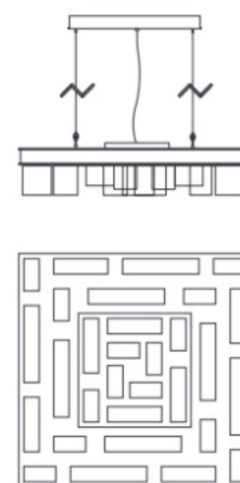
Item Gisele EX10 L.100 x D.100 cm H.45 cm min - 138 cm max
